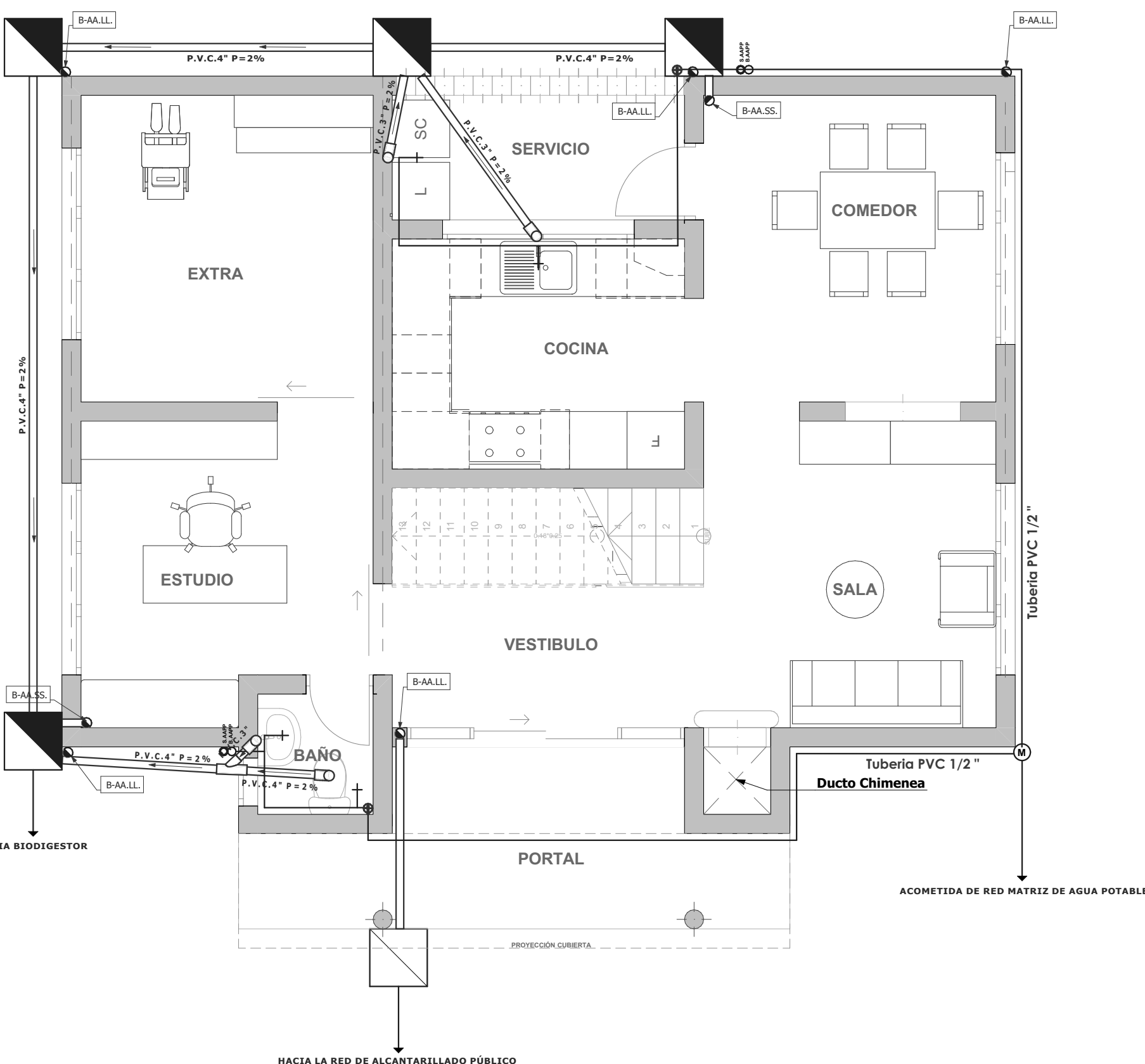
PLANTA BAJA | Esc 1:50
