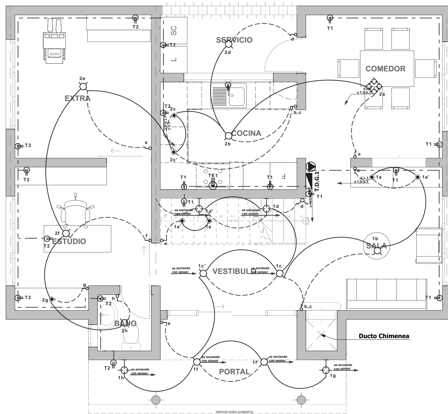
PLANTA BAJA | Esc 1:50
