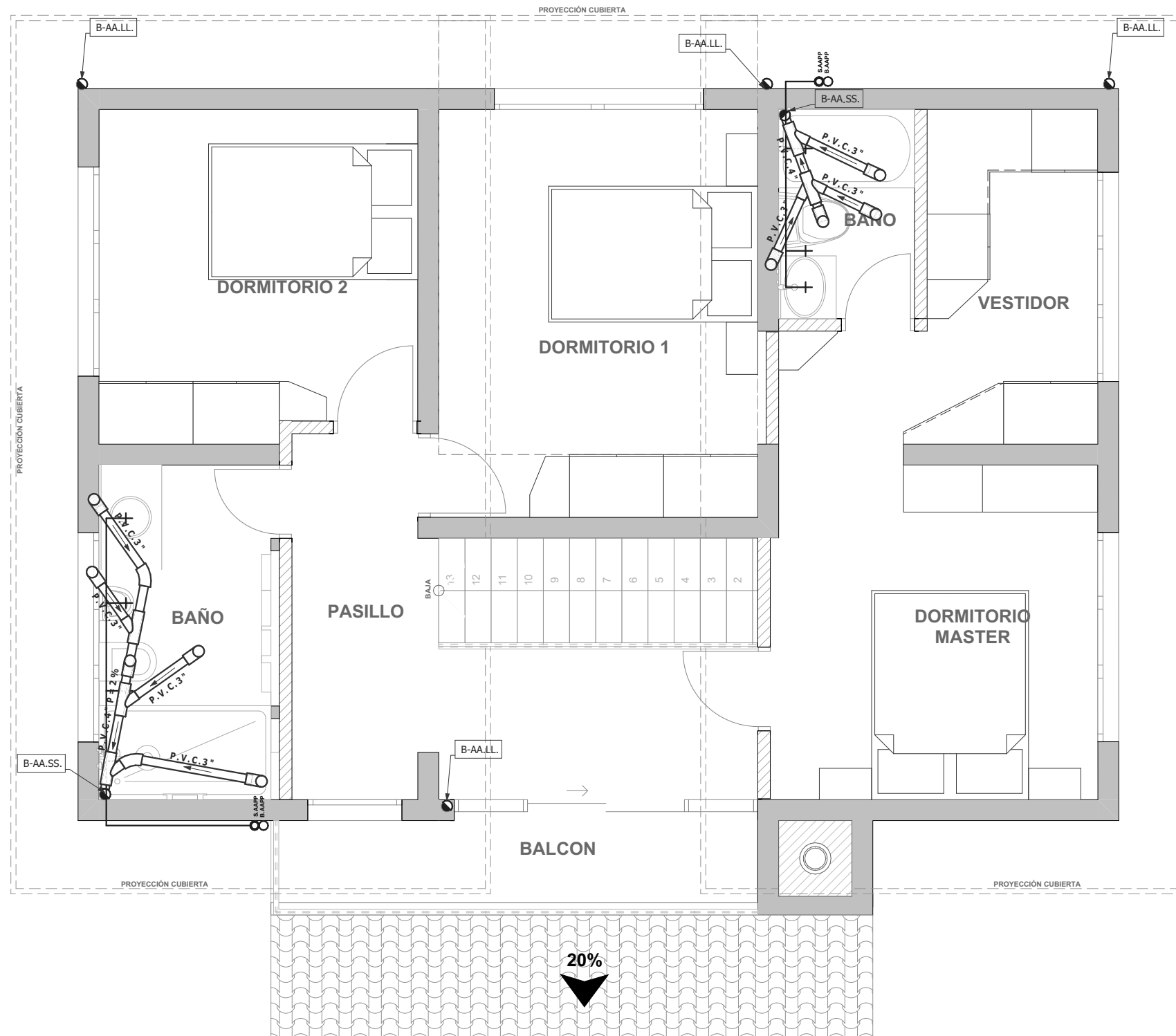
PLANTA ALTA I | Esc 1:50
